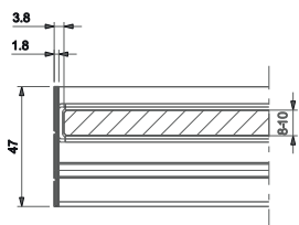
Standardausführung standard design
